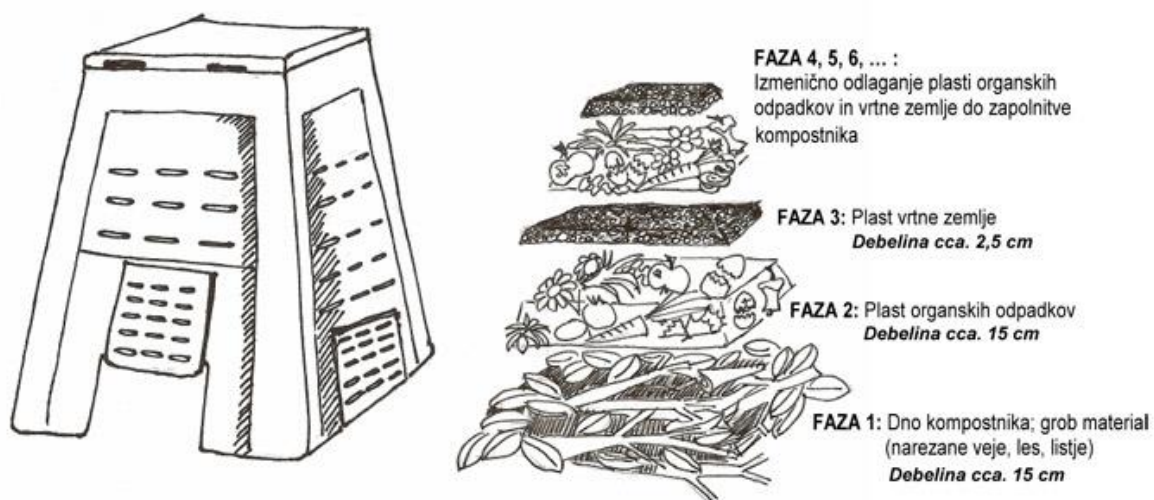
Slika 5 : Proces kompostiranja
